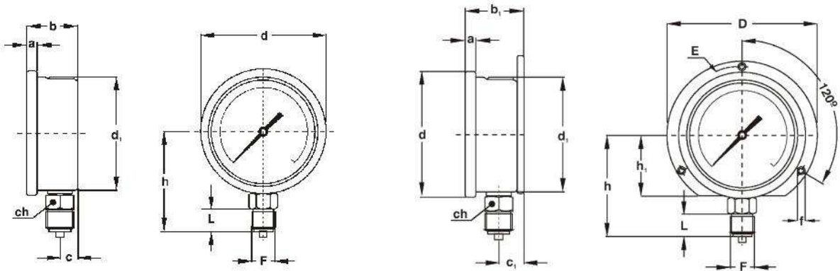
TYPE 1 Pour un montage local direct Con Raccord vertical
